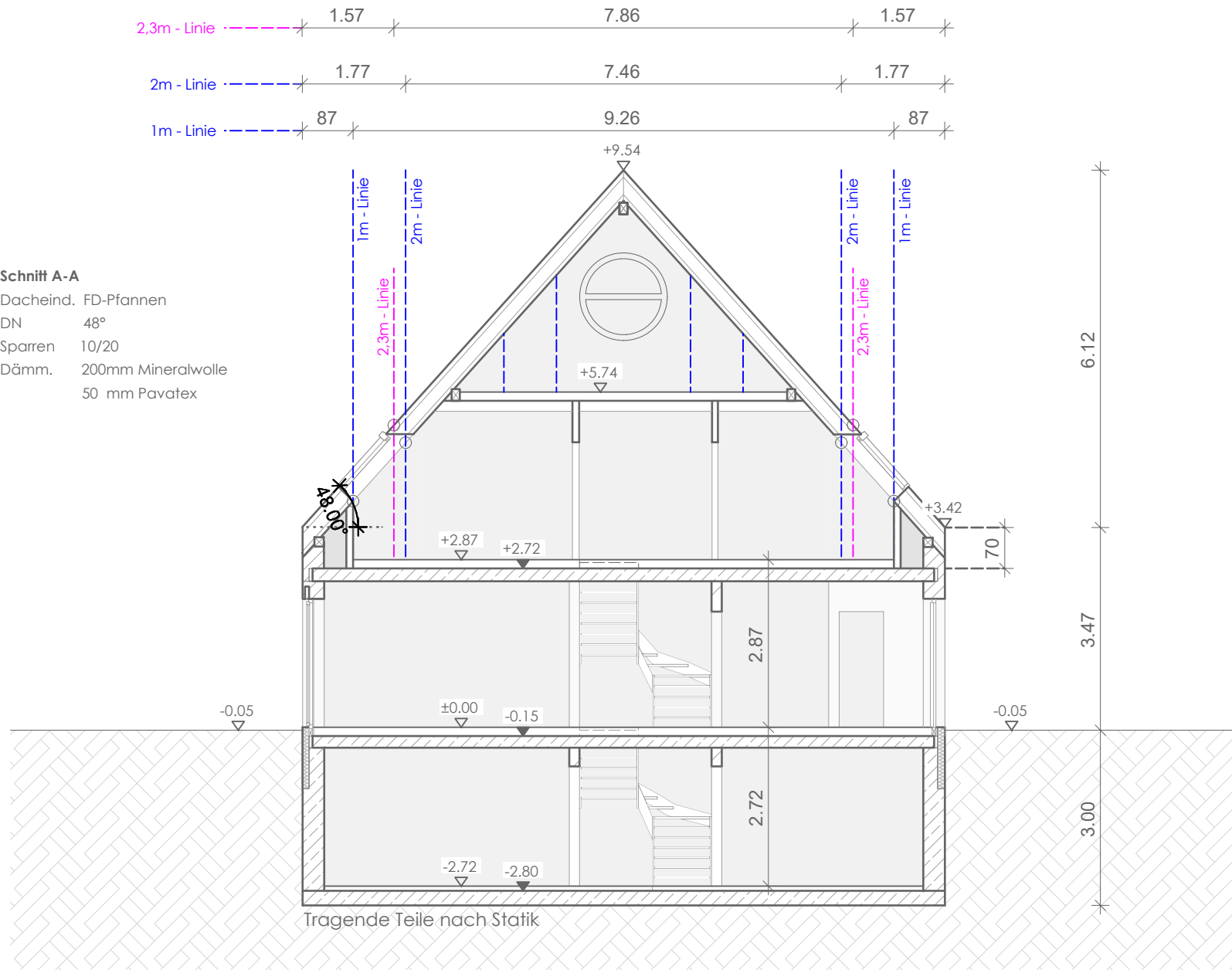
Schnitt A-A
